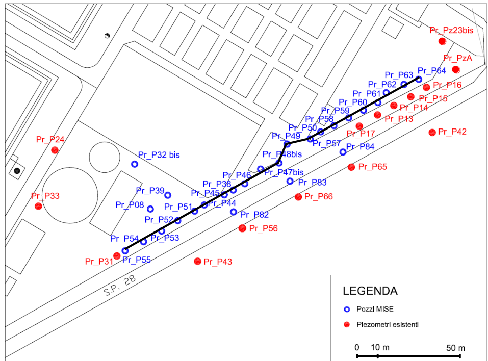
Figura 3.7.2 – Barriera di MISO
