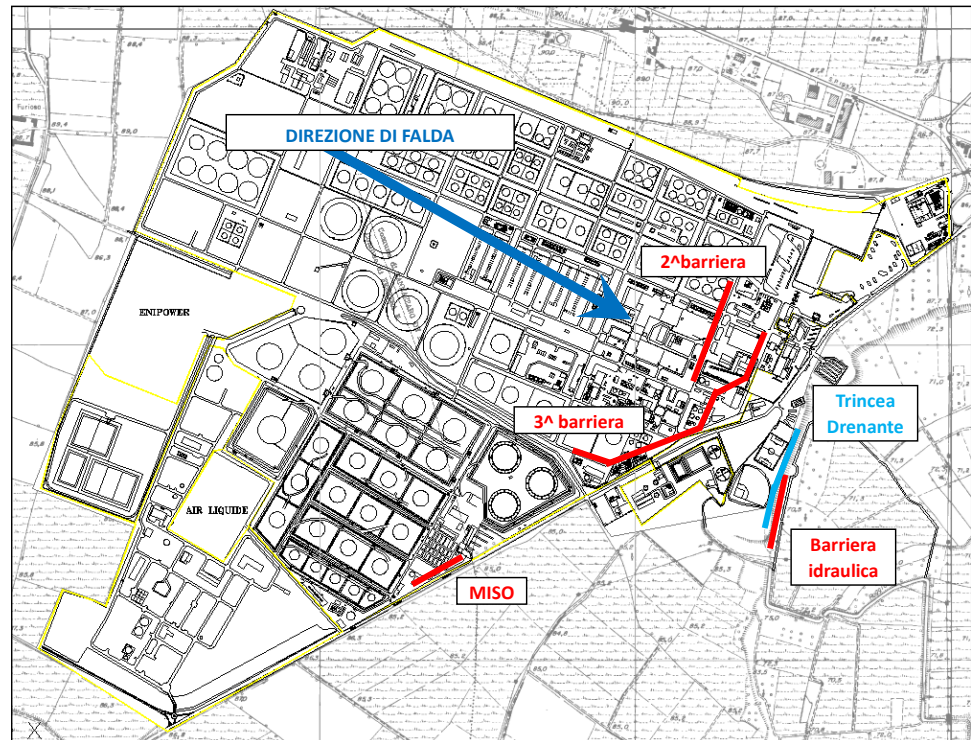
Figura 3.7.1 – Posizione delle barriere idrauliche
